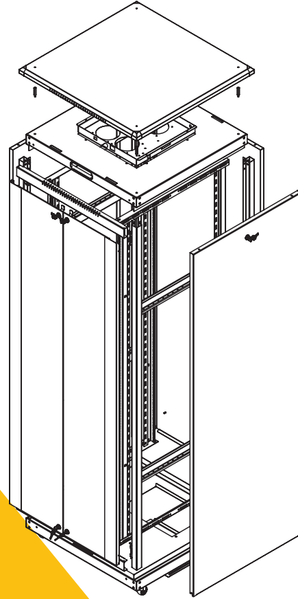
İZOMETRİK PATLATILMIŞ GÖRÜNÜŞ
